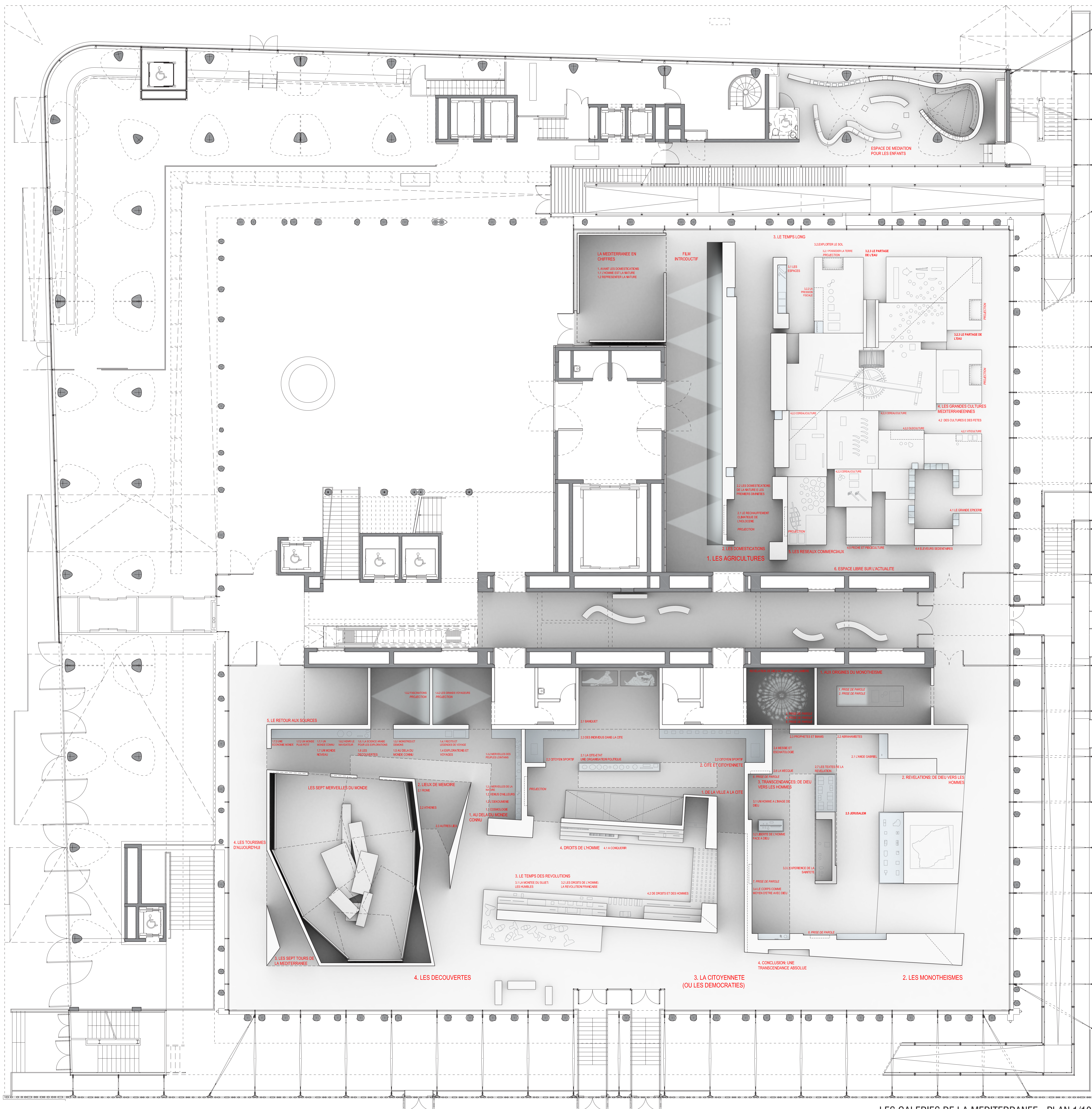
LES GALERIES DE LA MEDITERRANEE - PLAN 1/100
