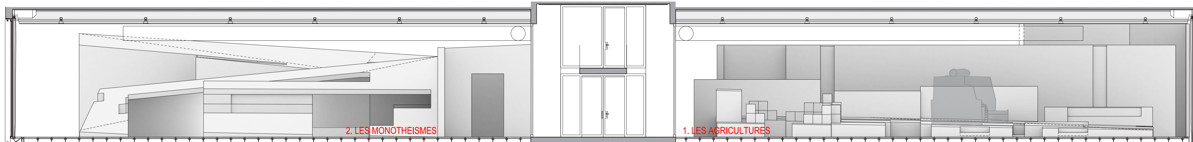
LES DEUX SALLES - COUPE 1/100
